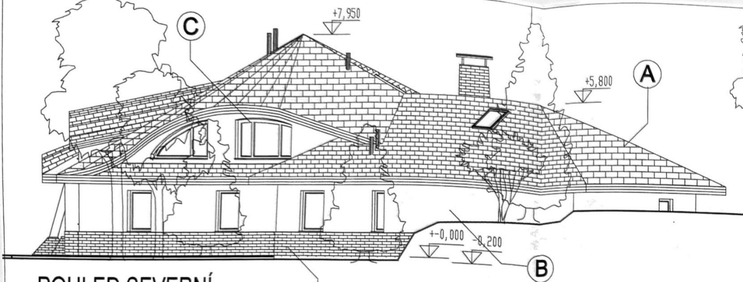
POHLED SEVERNÍ
