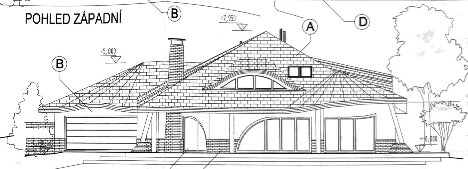
POHLED JIŽNÍ
